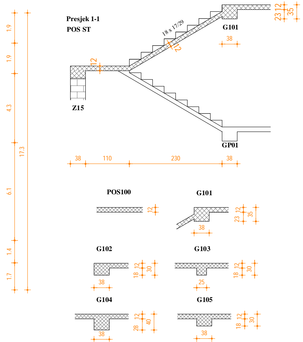
Detalji R 1:20 [cm]
