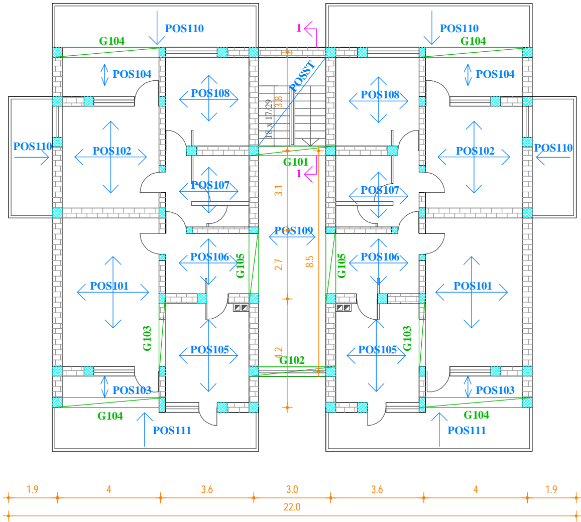
Plan pozicija u nivou tavanice POS100 - AB ploča R 1:50 [m]
